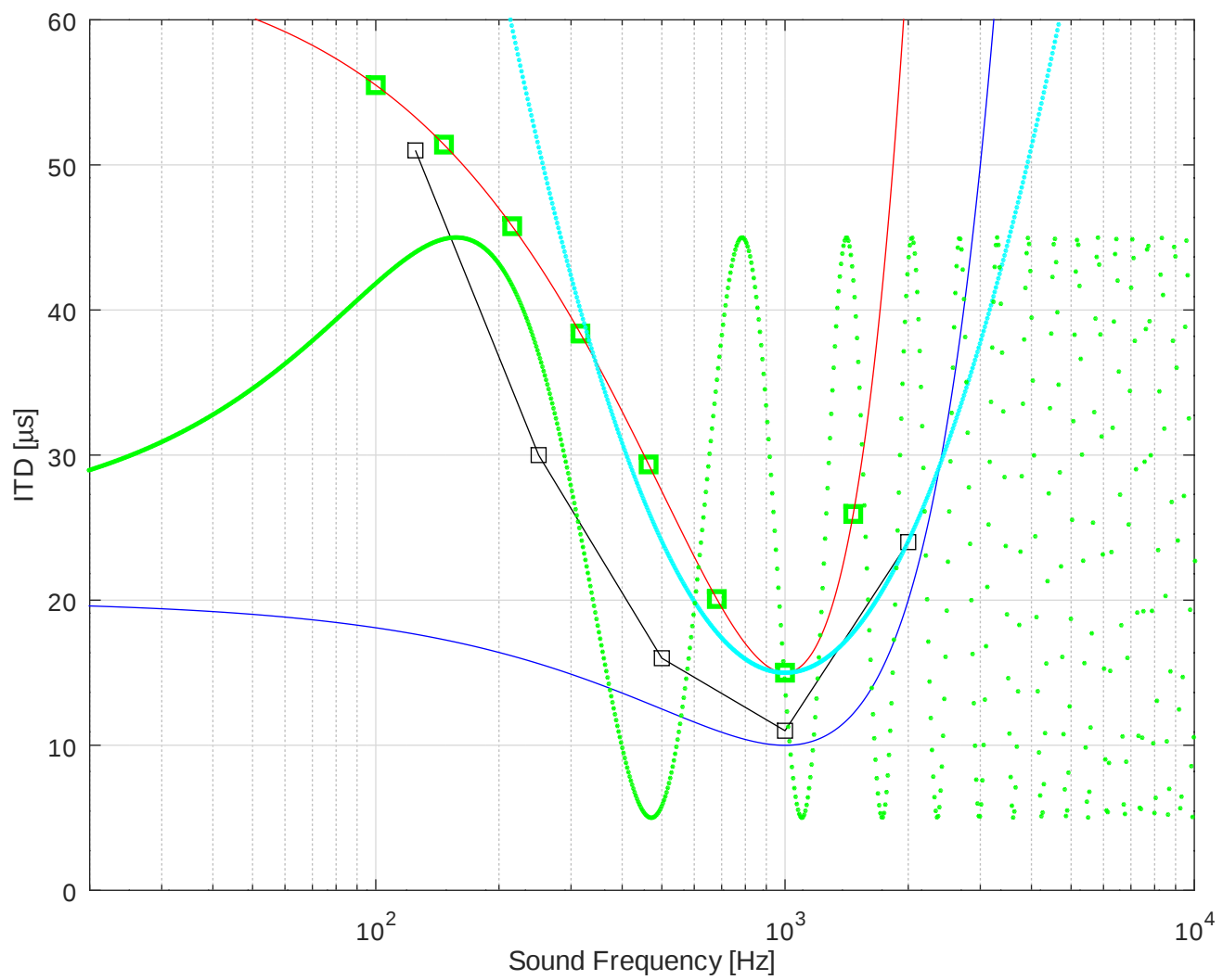
Fig.: FM2BV1.m
